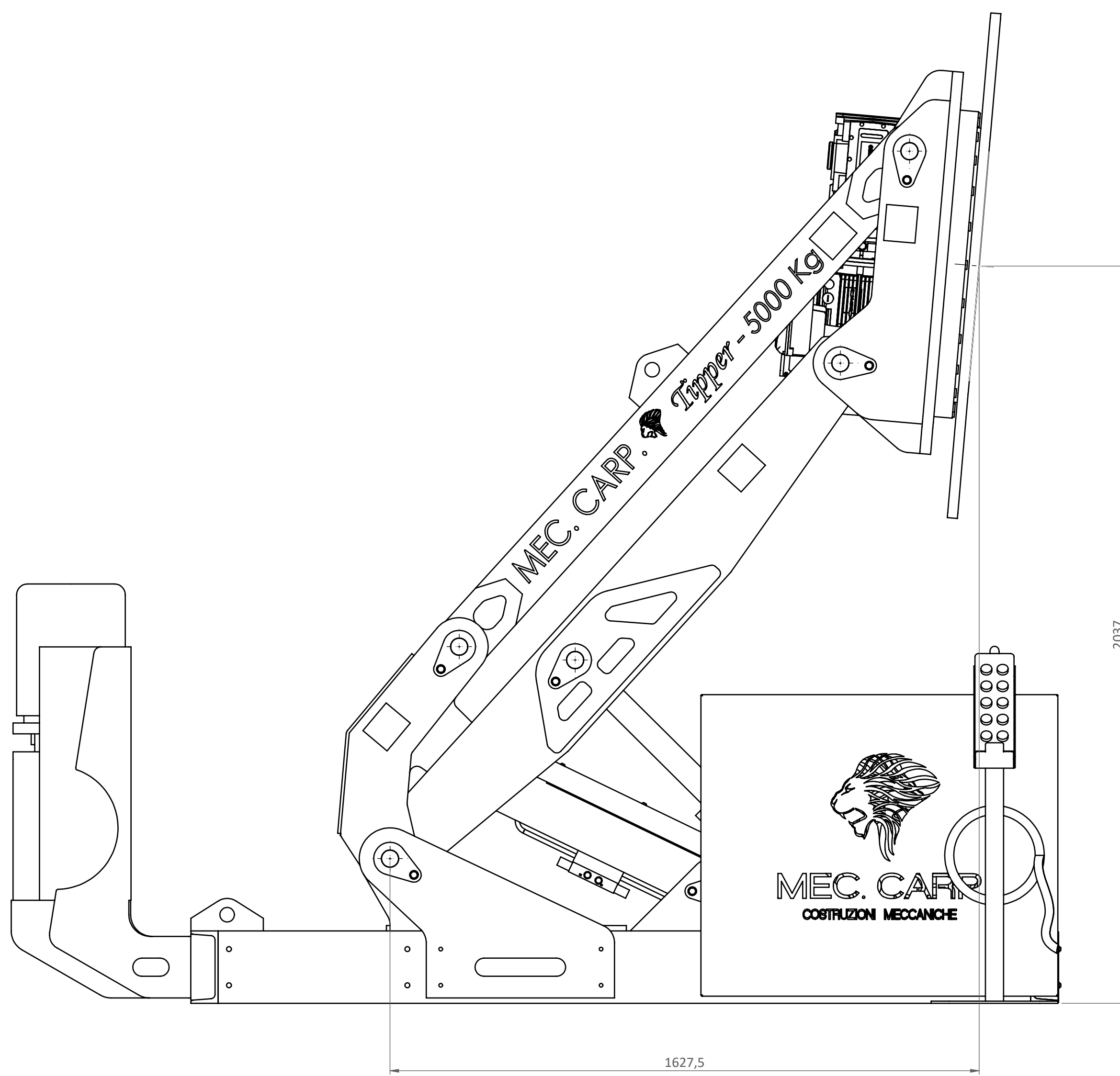
POSIZIONATORE ALTO TAVOLA A 95°
