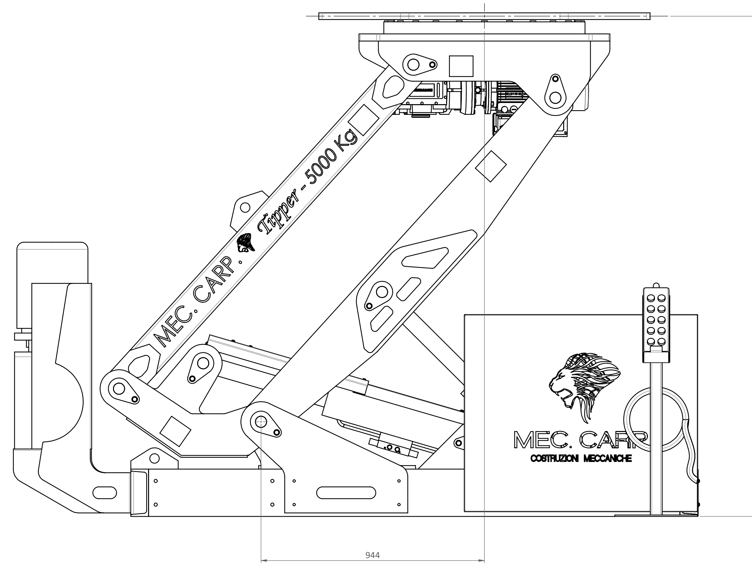
POSIZIONATORE ALTO TAVOLA A 0°
