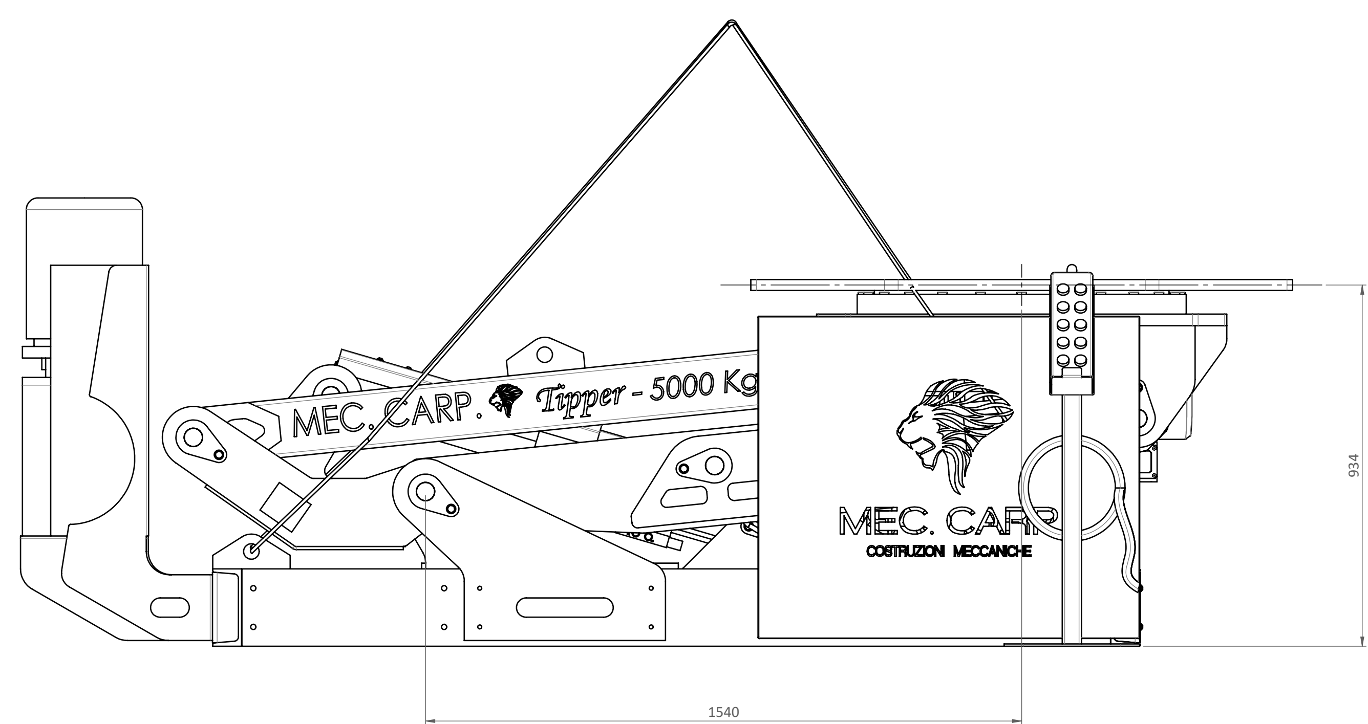
POSIZIONATORE BASSO TAVOLA A 0°
