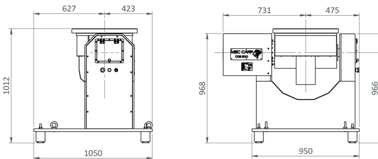
COB500 CON TAVOLA IN POSIZIONE ORIZZONTALE
