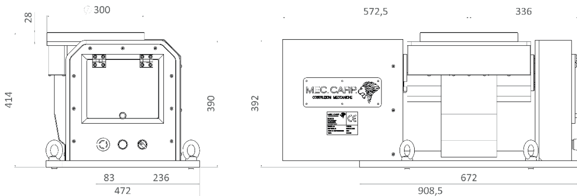
COB100 CON TAVOLA IN POSIZIONE ORIZZONTALE
