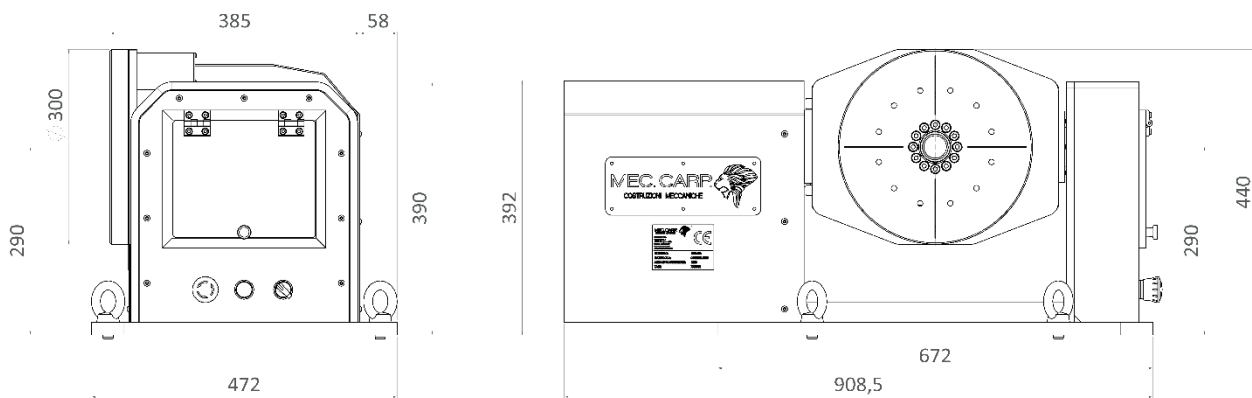
COB100 CON TAVOLA IN POSIZIONE ORTOGONALE
